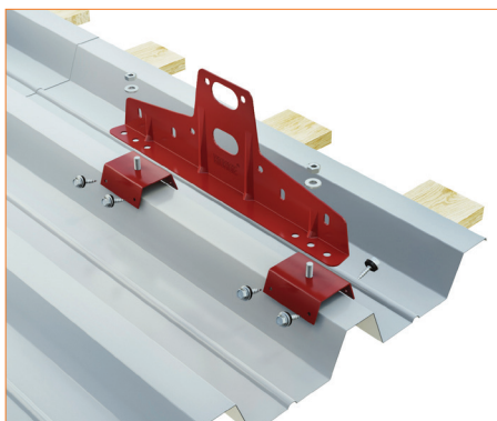
Снегозадержатель трубчатый для профнастила Н-60, Н-75, Н-114
